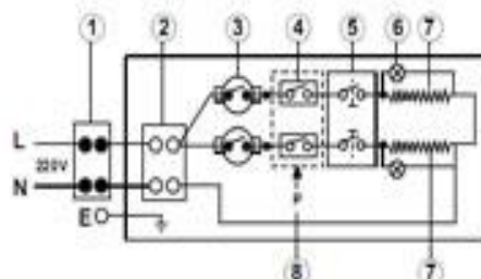
Водонагрівачи ATMOR мощністю від 7 до 9 кВт (однофазні)
