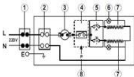
Водонагрівачи ATMOR мощністю до 6 кВт (однофазні)
