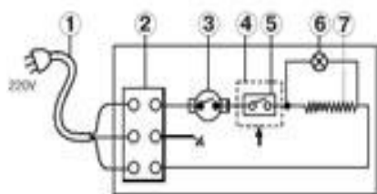
Водонагрівачи ATMOR мощністю до 3,5 кВт (однофазні)
